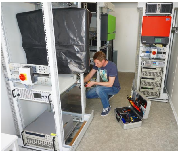
Aufbau der Teststände am KIT, mit denen die Sicherheit, Qualität und Netzdienlichkeit von Heimspeichern für Strom aus Photovoltaikanlagen analysiert wird (Foto: KIT).
